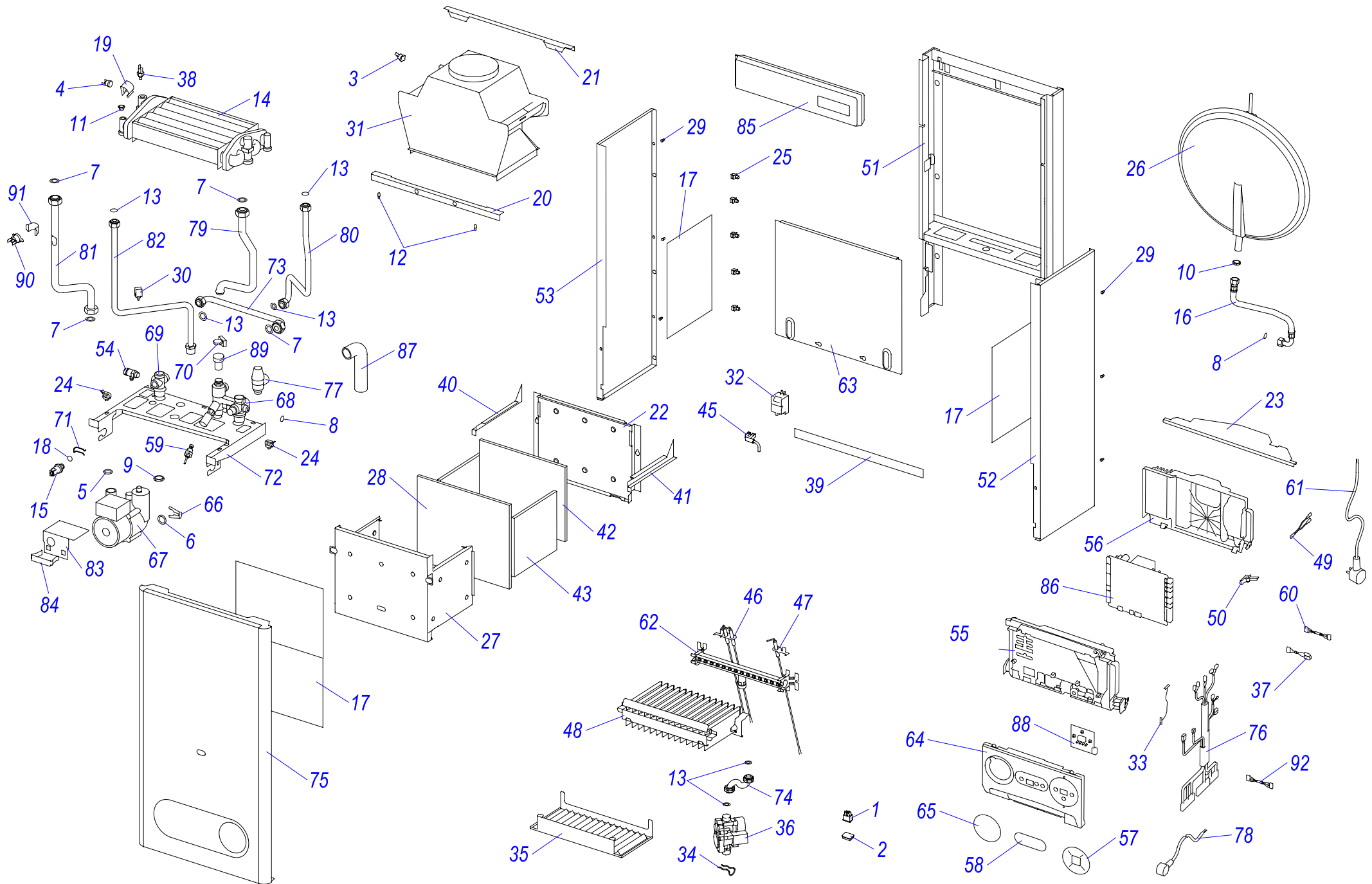
Навесные котлы
