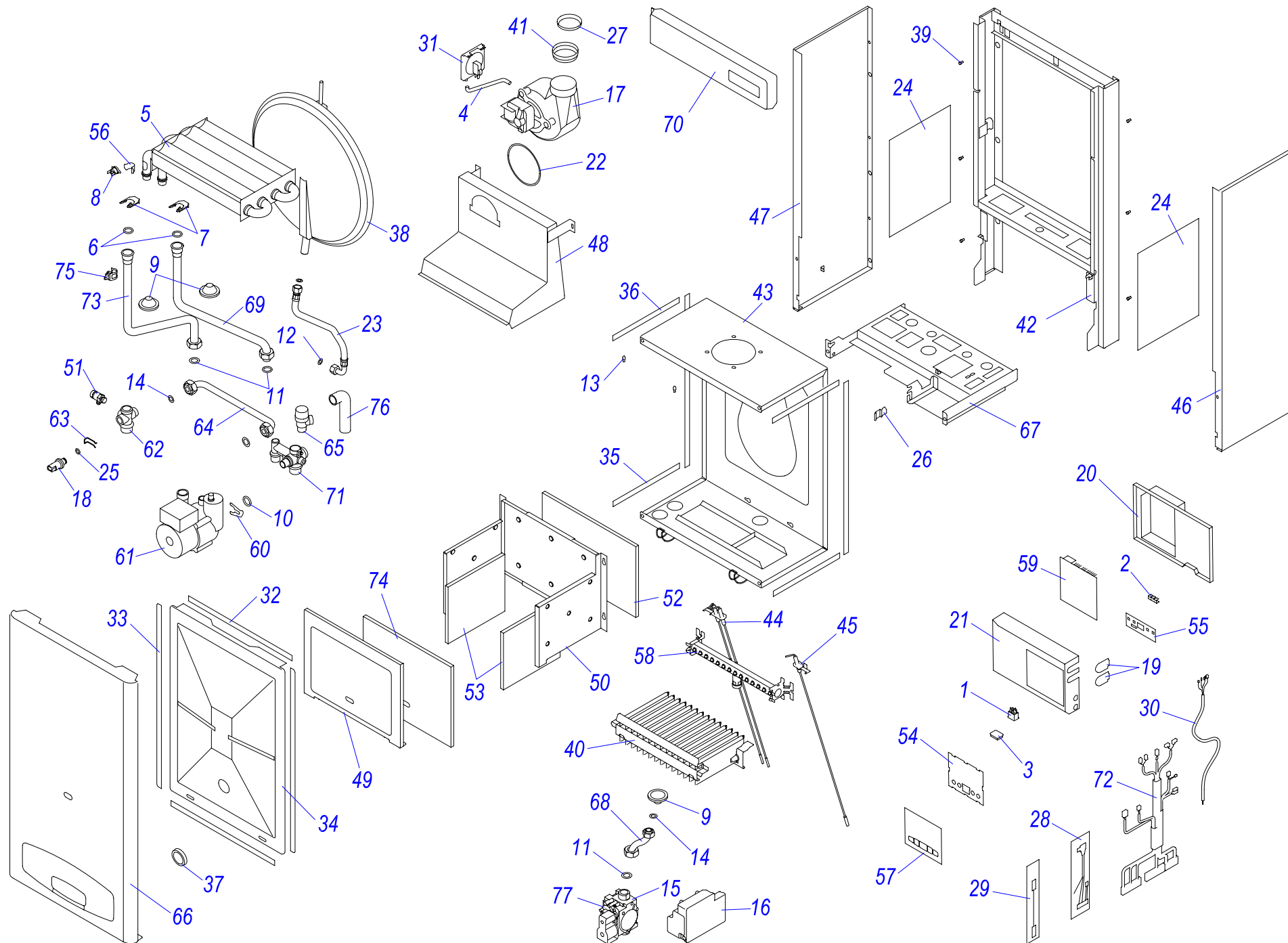
Навесные котлы
